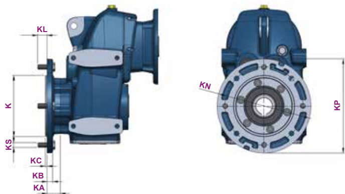
Kołnierz wyjściowy
